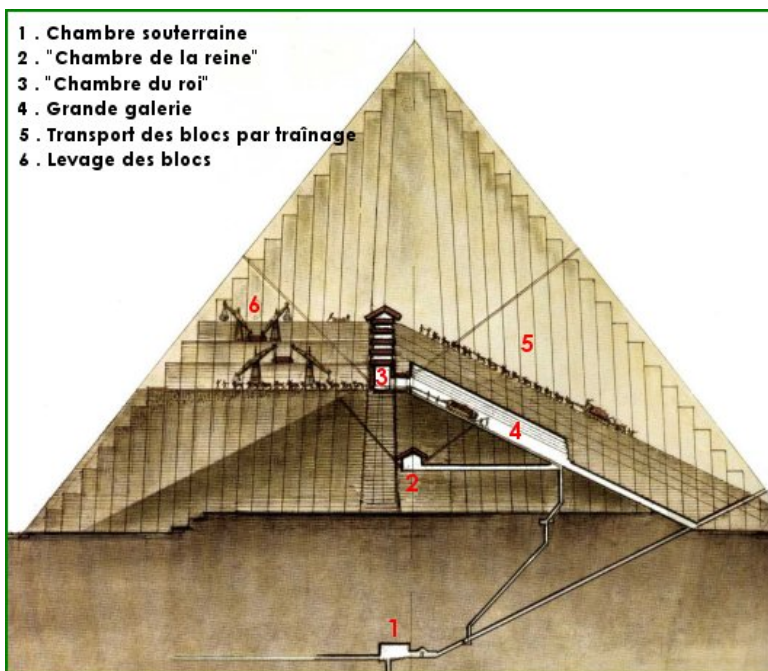
Coupe de la pyramide de Kheops
